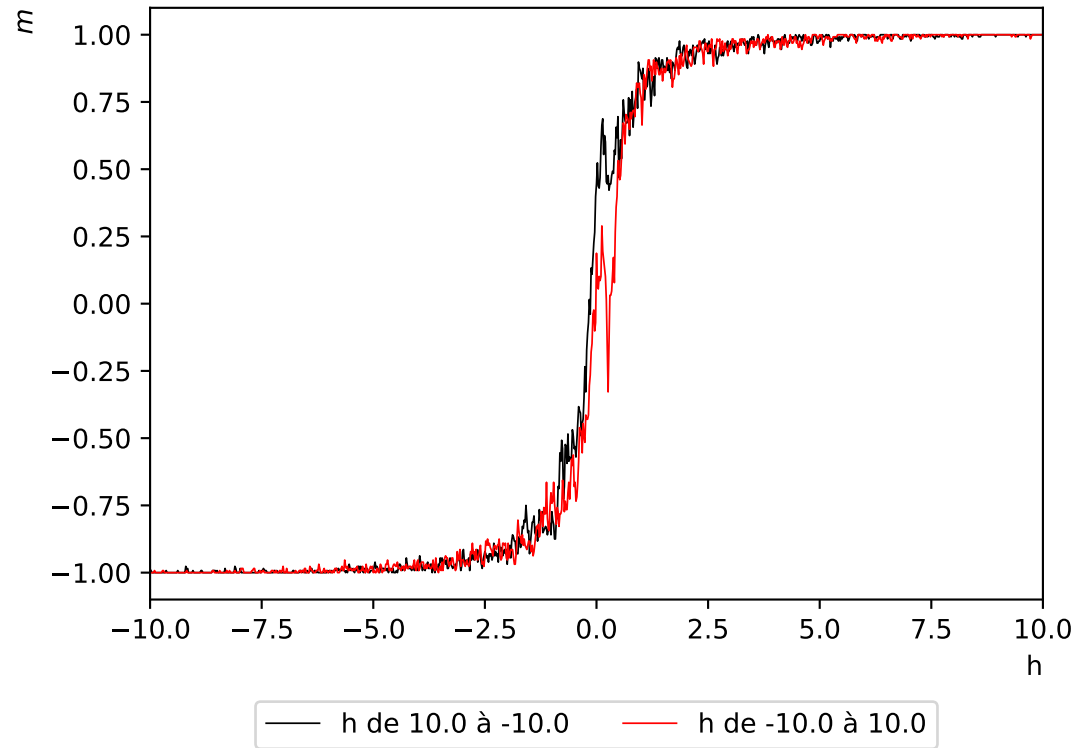
Hystérésis de l'aimantation - réseau de taille L=16 - champ magnétique d'amplitude h=10 à T=3.5
